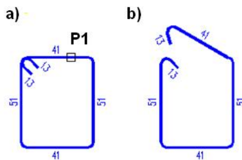
Rys. 1. Zwymiarowane strzemię: a) przed otwarciem, b) po otwarciu
