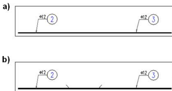
Rys. 1. Pręty proste bez haków w płaszczyźnie prostopadłej do rysunku: a) bez znaczników końca pręta, b) ze znacznikami
