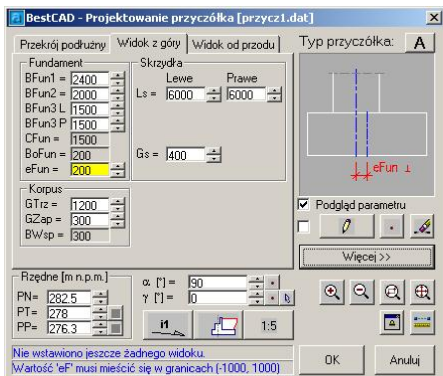
Rys. 1. Okno dialogowe Projektowanie przyciółka –Widok z góry
