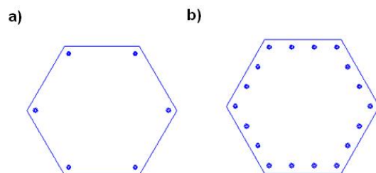
Rys. 3. Przekrój słupa: a) ze zbrojeniem w narożach, b) ze zbrojeniem w narożach i prętami pośrednimi
