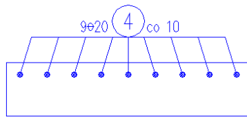
Rys. 1. Opis symetryczny prętów
