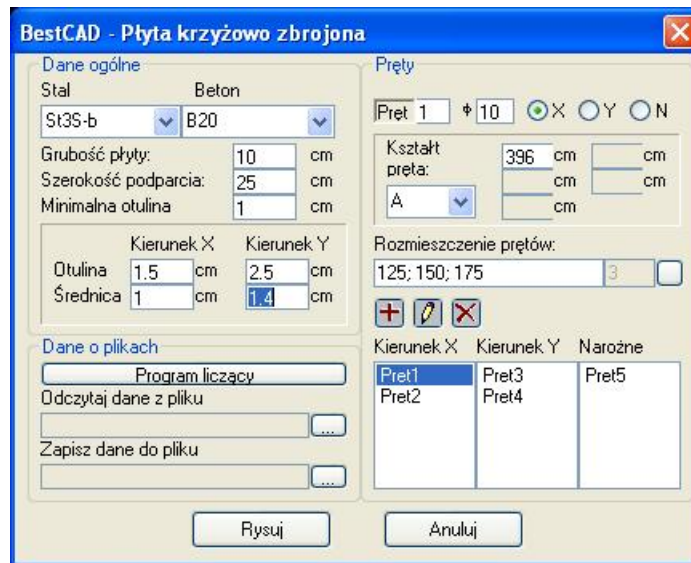
Rys. 1. Okno dialogowe Płyta krzyżowo zbrojona
