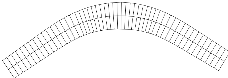
Rys. 3. Przykład gotowego rysunku – poszerzenie na łuku z krzywymi przejściowymi
